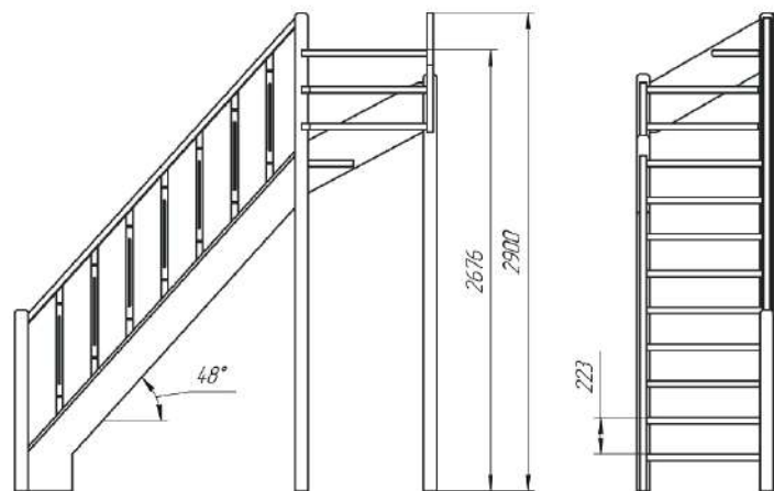
Рисунок 1. Лестница внутриквартирная ЛЕС-715.
